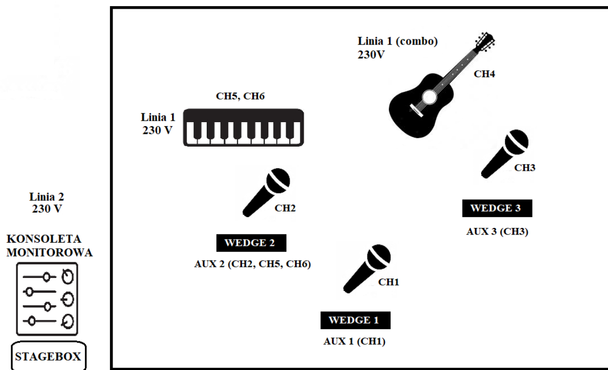
Rysunek 1. Plan sceny dla dźwięku
