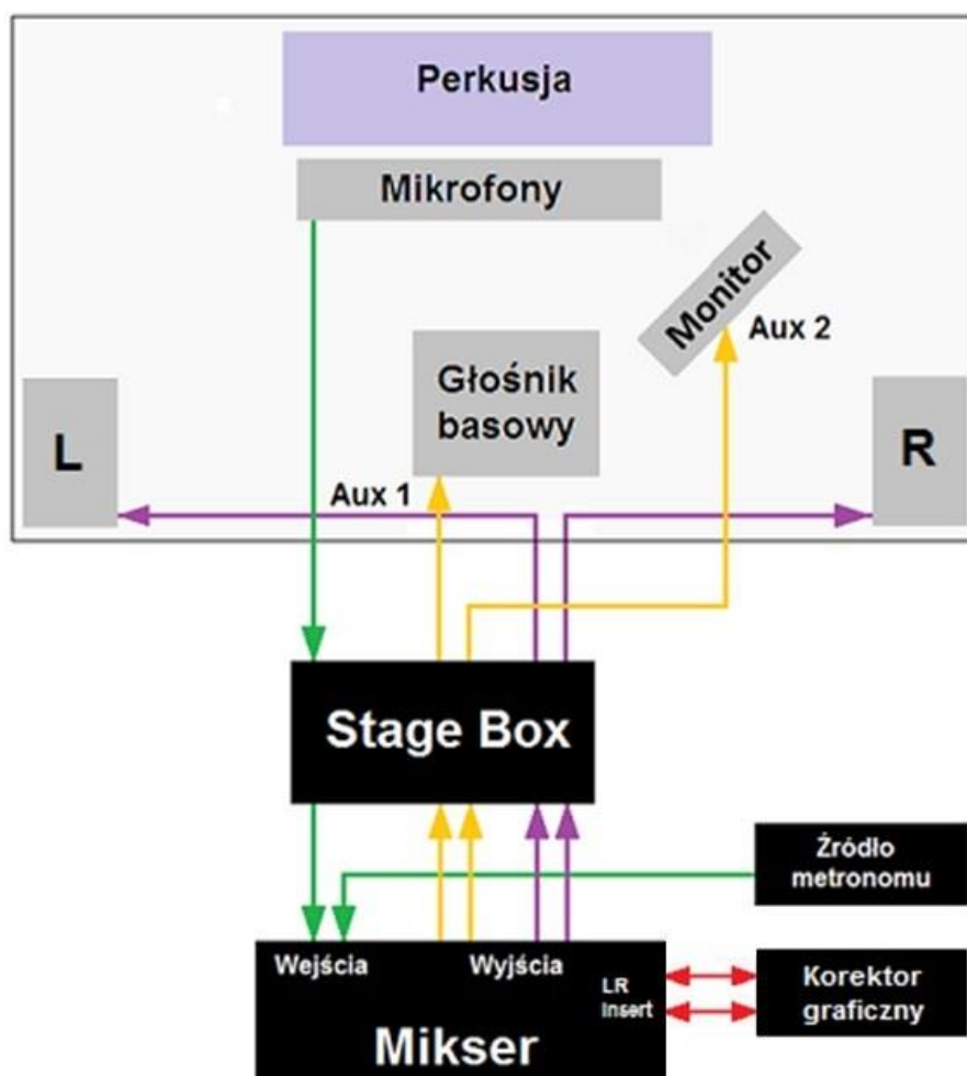
Rysunek 1. Schemat systemu elektroakustycznego
