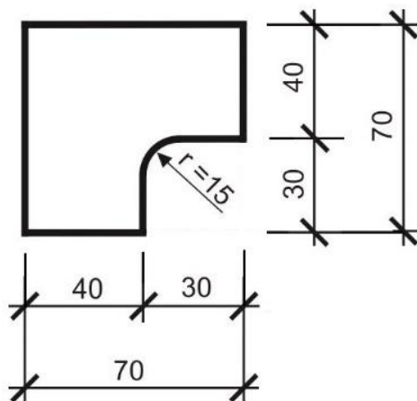
Rys. 4. Wzór szablonu zaokrąglenia krawędzi parapetu
