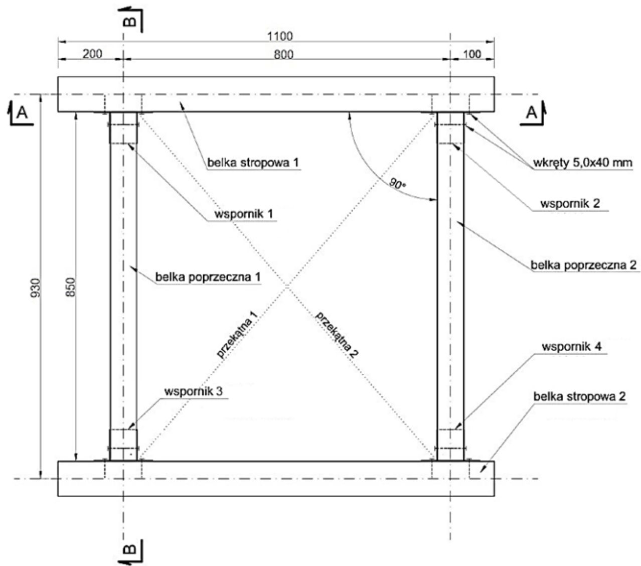
Rysunek 1. Fragment konstrukcji stropu drewnianego – widok z góry
