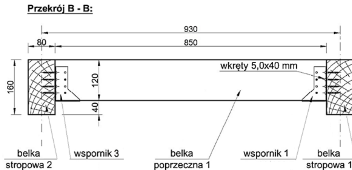
Rysunek 2. Fragment konstrukcji stropu drewnianego – przekroje A-A i B-B
