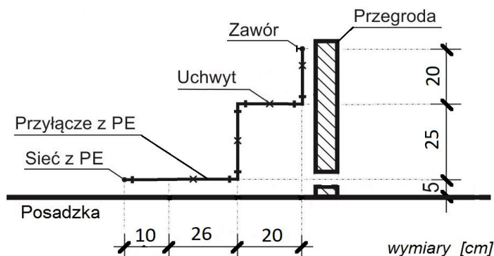
Rysunek 1. Przekrój pionowy przyłącza wodociągowego
