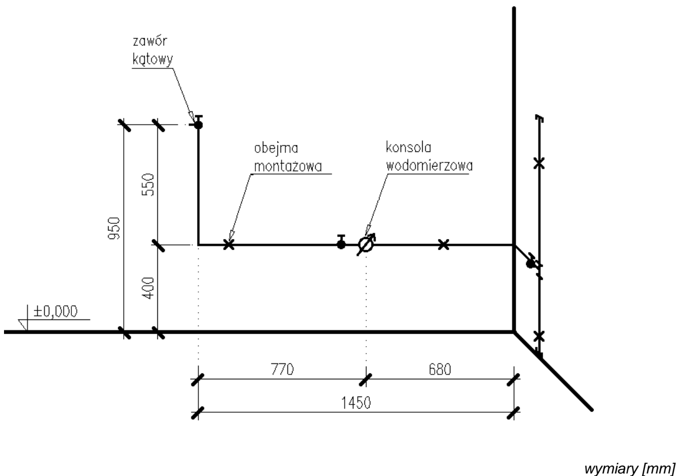
Rysunek 1. Widok instalacji wodociągowej
