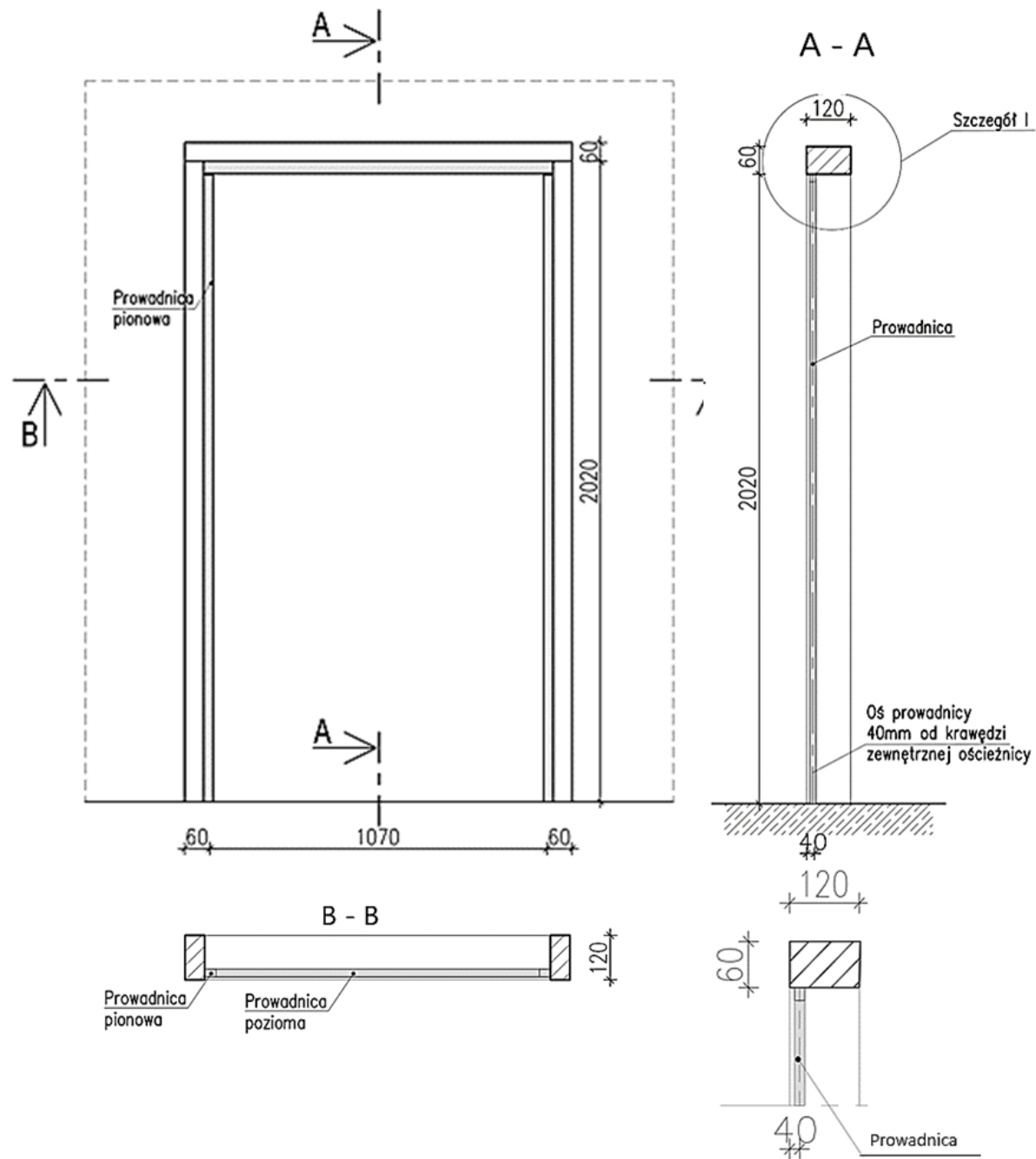
Ościeżnica z zamocowanymi przewodnikami
