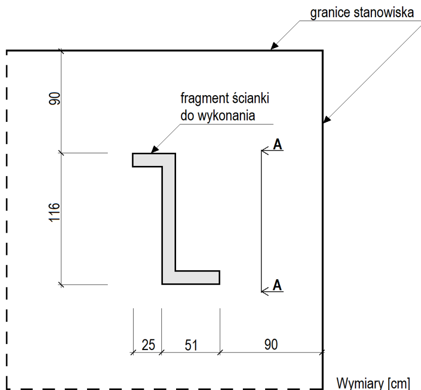
Rysunek 1. Usytuowanie fragmentu ścianki działowej na stanowisku egzaminacyjnym (rzut)
