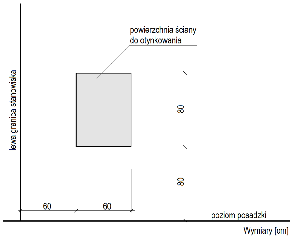
Rysunek 4. Usytuowanie powierzchni tynku cienkowarstwowego na ścianie (widok)
