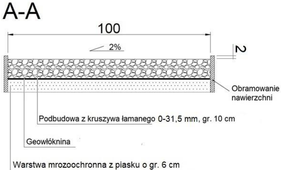
Rysunek 2. Przekrój poprzeczny nawierzchni (wymiarów podano w cm)
