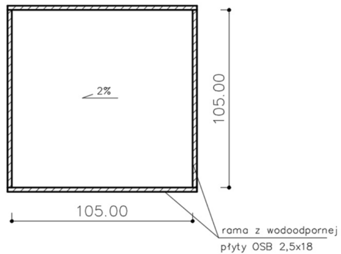
Rysunek 2. Rzut koryta
