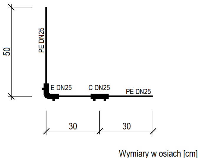
Rysunek 1. Fragment gazociągu z rur PE DN25
