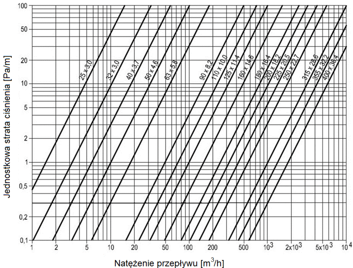
Rysunek 3. Nomogram do doboru średnic dla gazociągów niskiego ciśnienia PE100 SDR11
