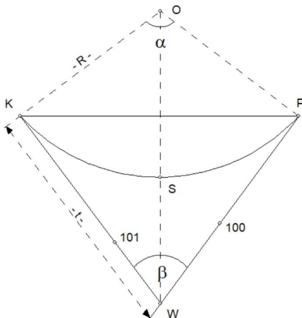
Rysunek 1. Szkic rozmieszczenia punktów łuku kołowego i punktów 100 i 101.
