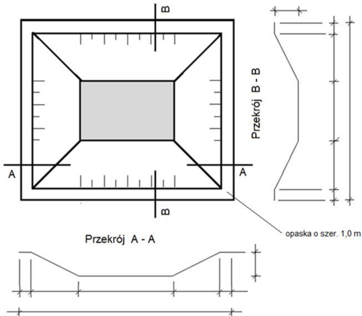
Rysunek 1. Przekroje poprzeczne zbiornika do zwymiarowania i opisanie wielkości nachylenia skarp
