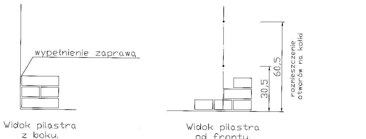
Rysunek 1. Istniejąca baza pilastra
