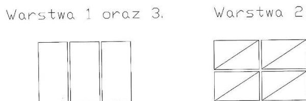
Rysunek 2. Układ cegieł w warstwach bazy pilastra
