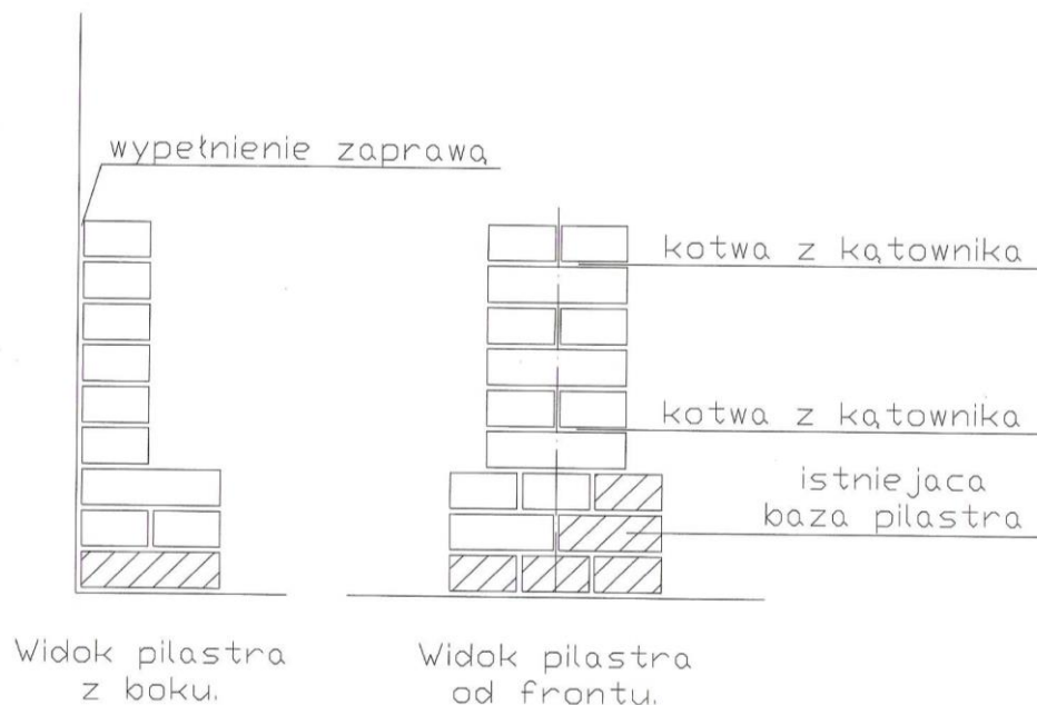
Rysunek 3. Widok pilastra po naprawie
