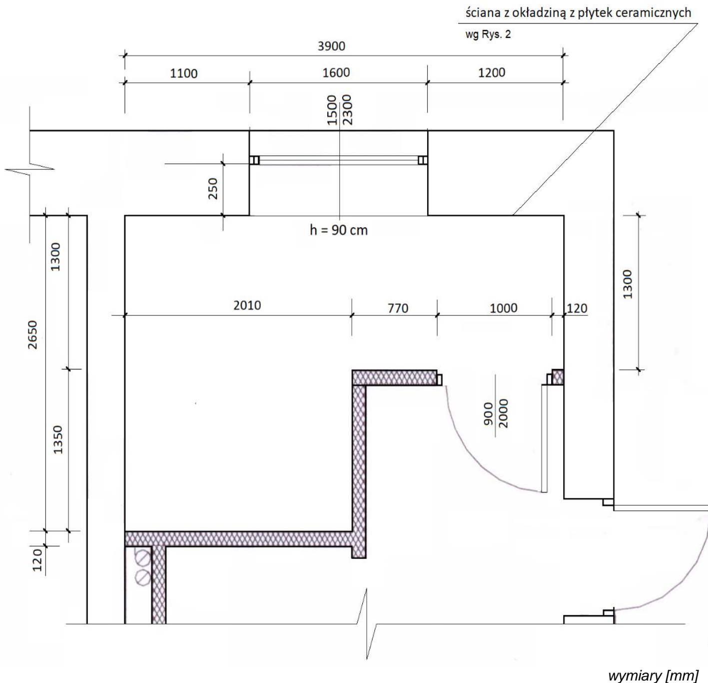
Rysunek 1. Rzut łazienki
