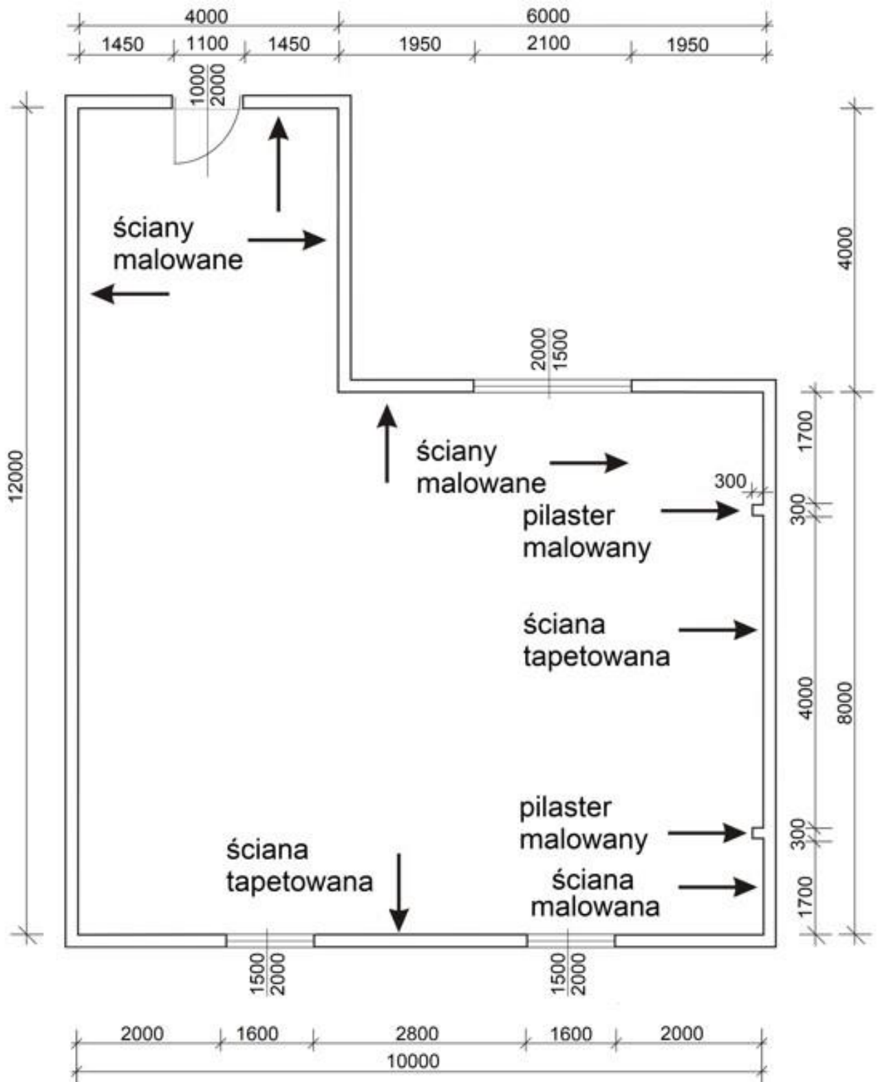
Rysunek 2. Rzut pomieszczenia wystawowego – wykończenie ścian
