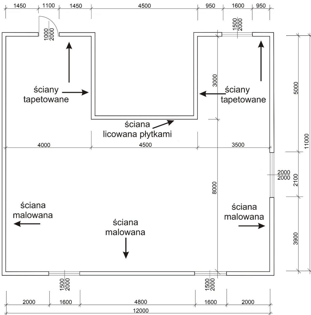
Rzut pomieszczenia kawiarni
