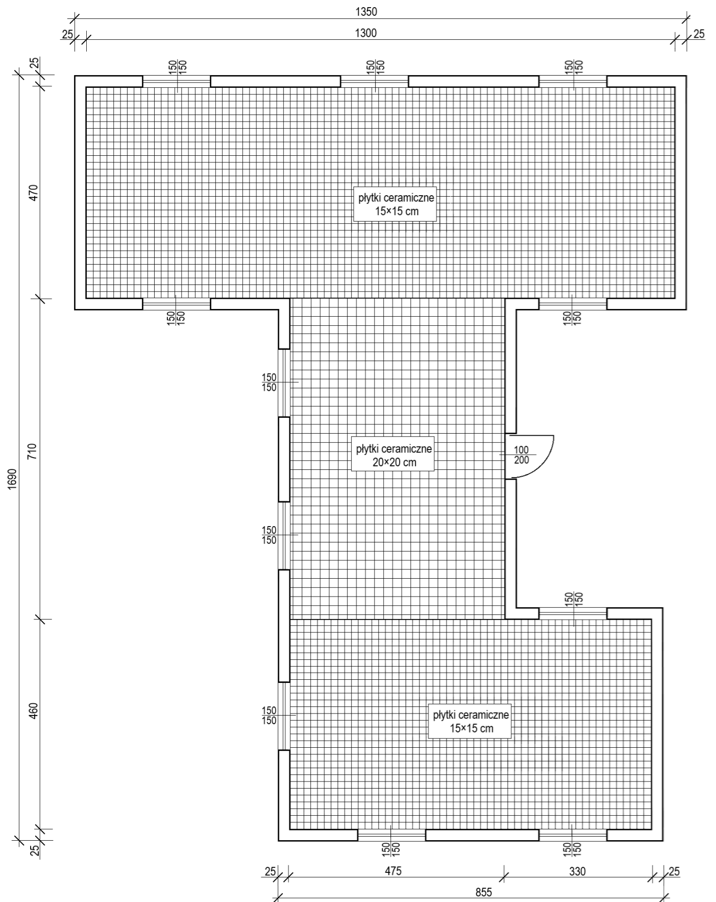
Rysunek 1. Rzut parteru – układ płytek na posadzkach
