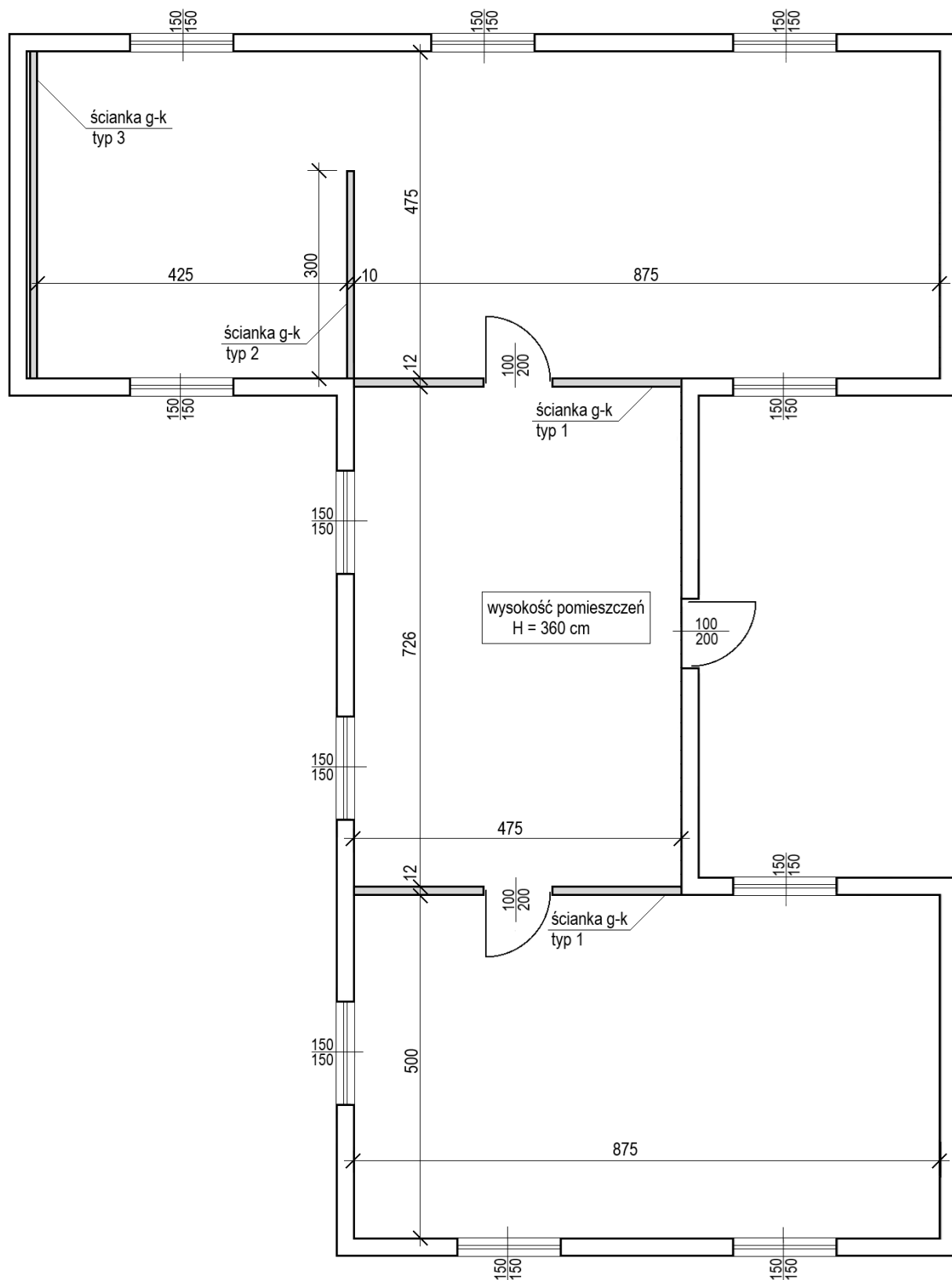
Rysunek 2. Rzut parteru – usytuowanie ścianek działowych
