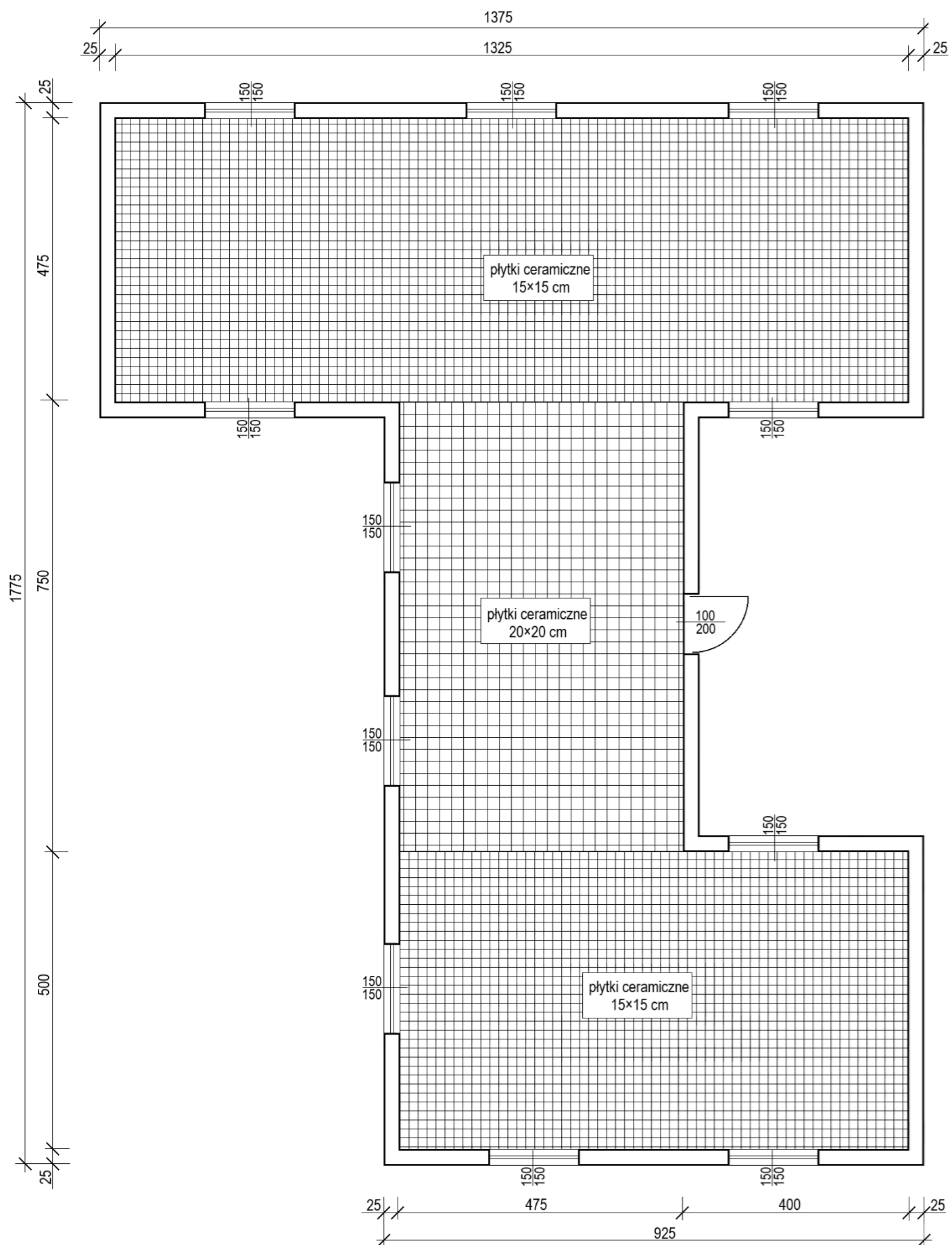
Rysunek 1. Rzut parteru – układ płytek na posadzkach
