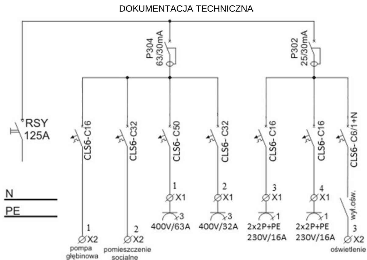
Rysunek 1. Schemat rozdzielnic RB1
