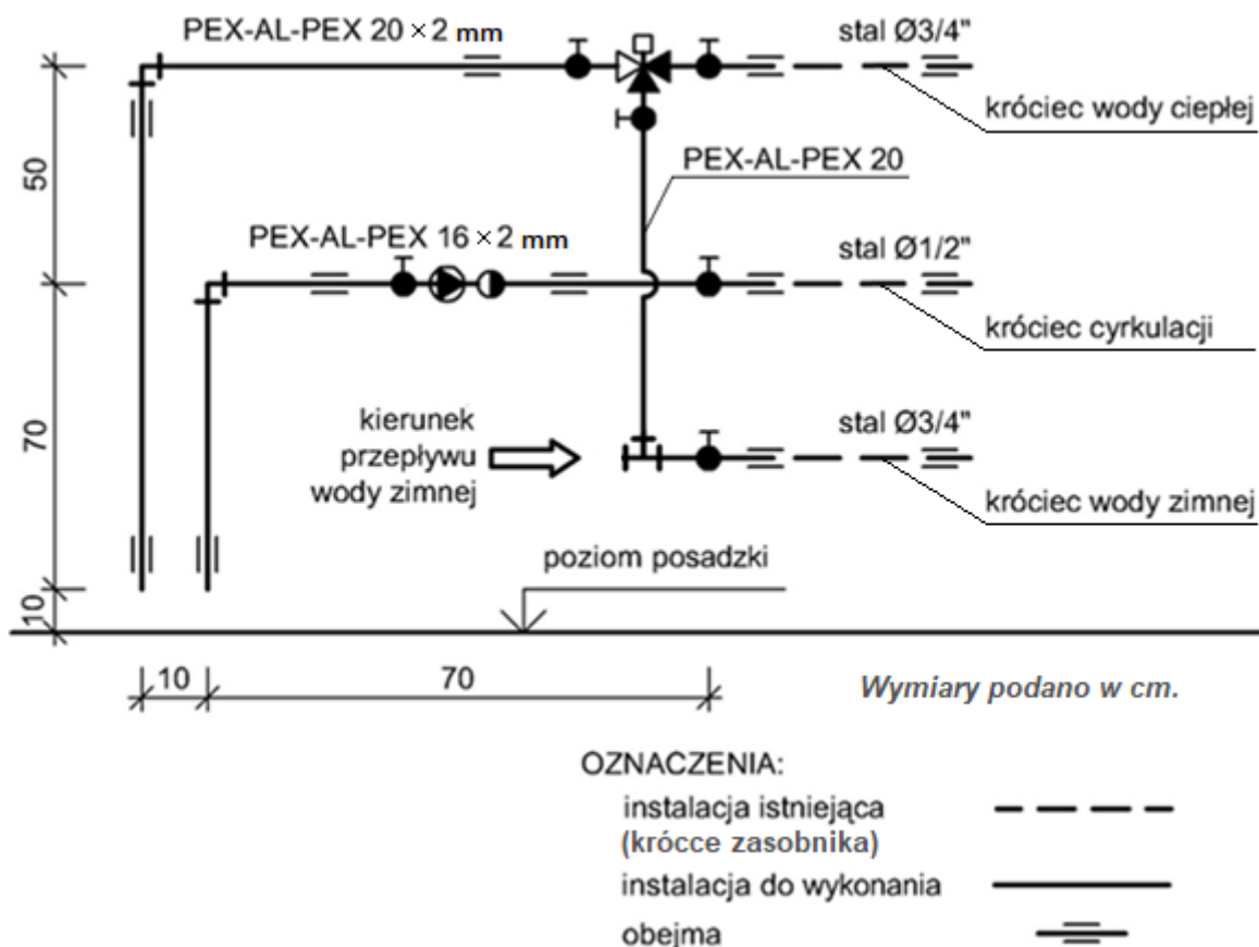
Rysunek 1. Podłączenie instalacji wody zimnej i ciepłej wody użytkowej wraz z przewodem cyrkulacyjnym do króćców zasobnika solarnego
