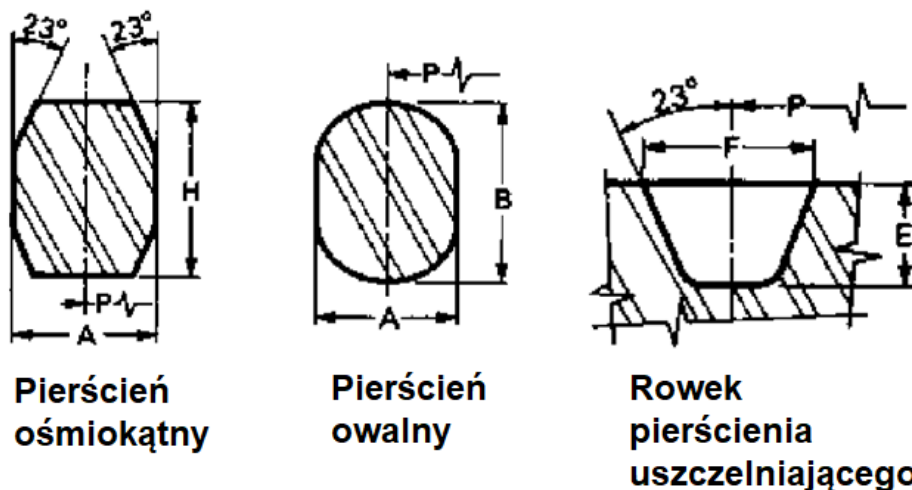
Rysunek 3. Schematy przekroju pierścieni uszczelniających i rowka
