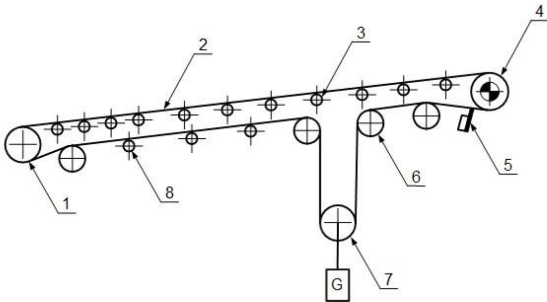
Rysunek 3. Budowa przenośnika taśmowego
