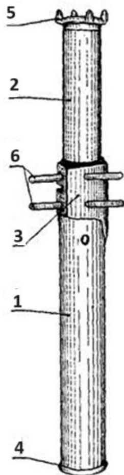
Rysunek 2. Stojak cierny typu Valent
