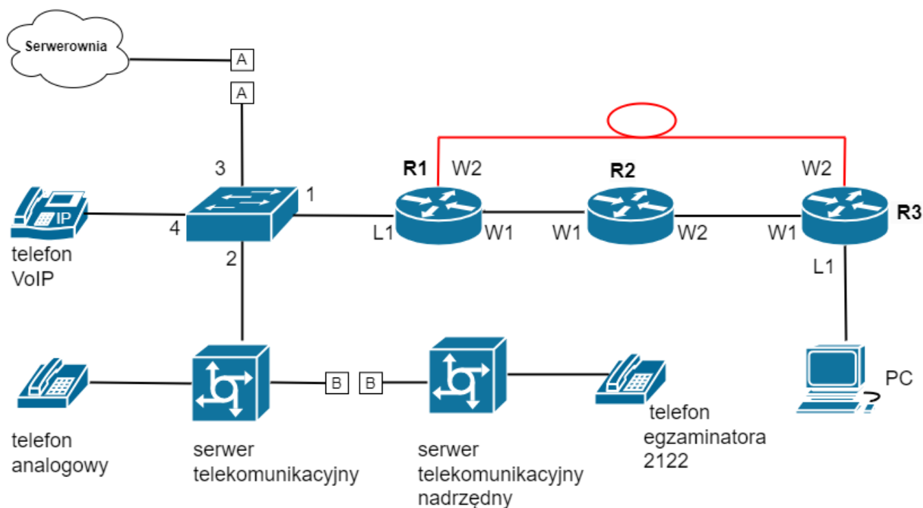
Schemat sieci teleinformatycznej
