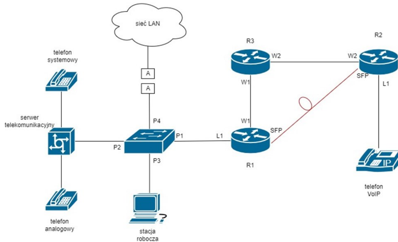
Schemat sieci teleinformatycznej
