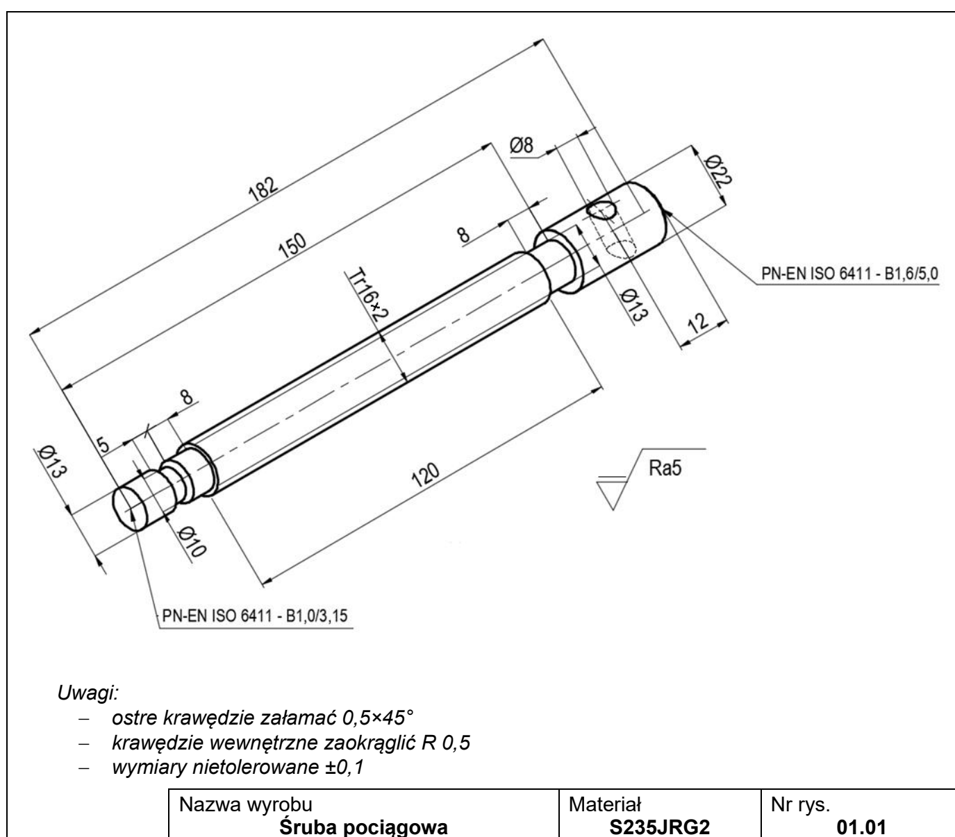
Rysunek 1. Śruba pociągowa
