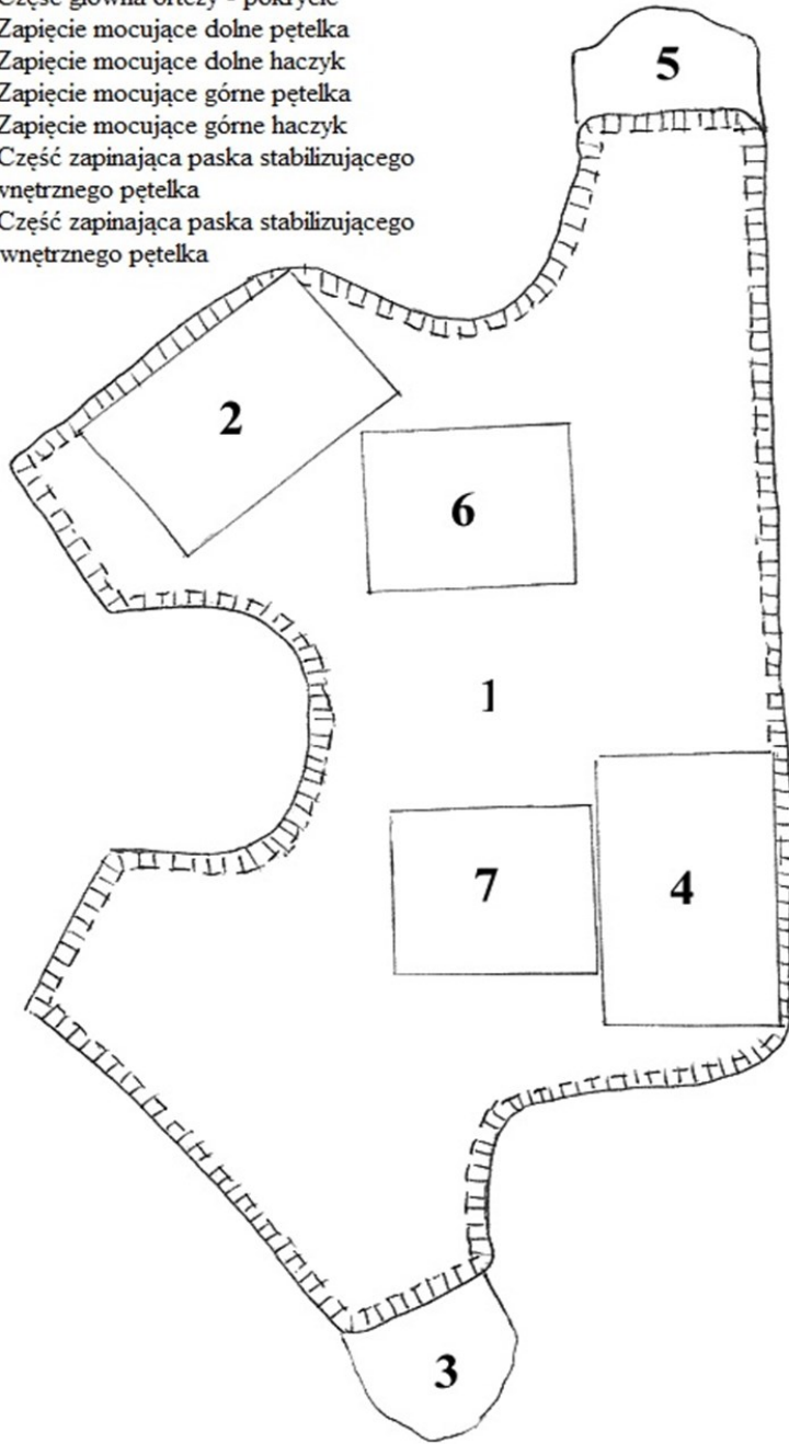
Rysunek 1. Orteza w rozłożeniu – wierzch
