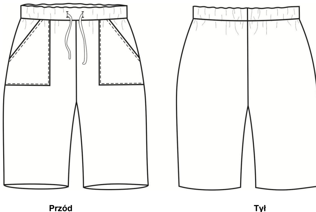
Rysunek modelowy spodni damskich
