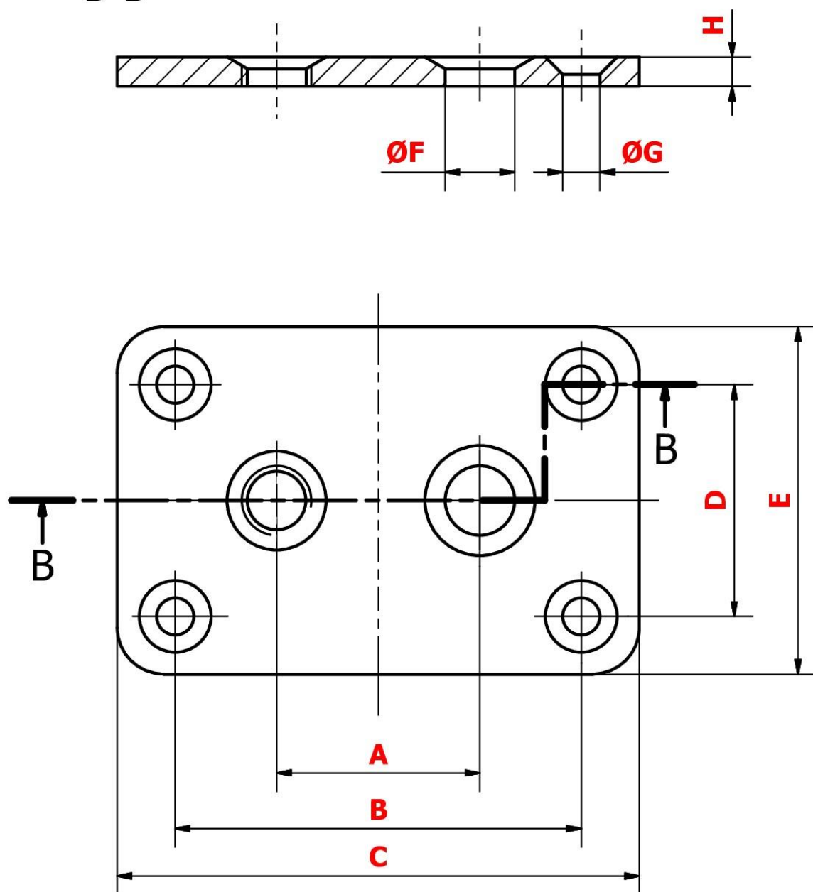
Rysunek 2. Wymiary płytki do obijania i wyciągania modelu
