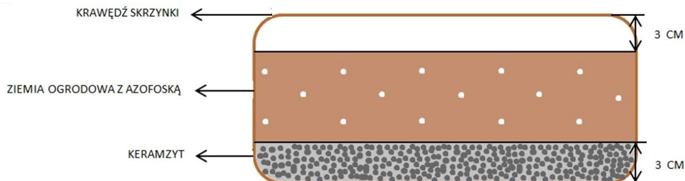
Rysunek 3. Przekrój poprzeczny skrzynki
