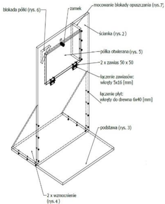
Rys. 1. Model ścianki nośnej z otwieraną półką.
